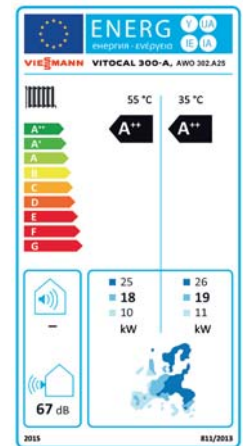
Energieeffizienzlabel Vitocal 300-A, AWO 302.A25
